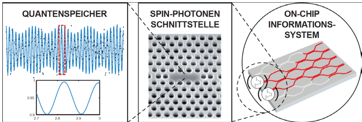
Bild 2: Prinzipische Skizze zu photonischen Schaltkreisen in Diamant. Die Quantenspeicher in Diamant werden auf einem Chip mit photonischen Elementen wie Wellenleitern verbunden. (Quelle: Humboldt-Universität zu Berlin)
